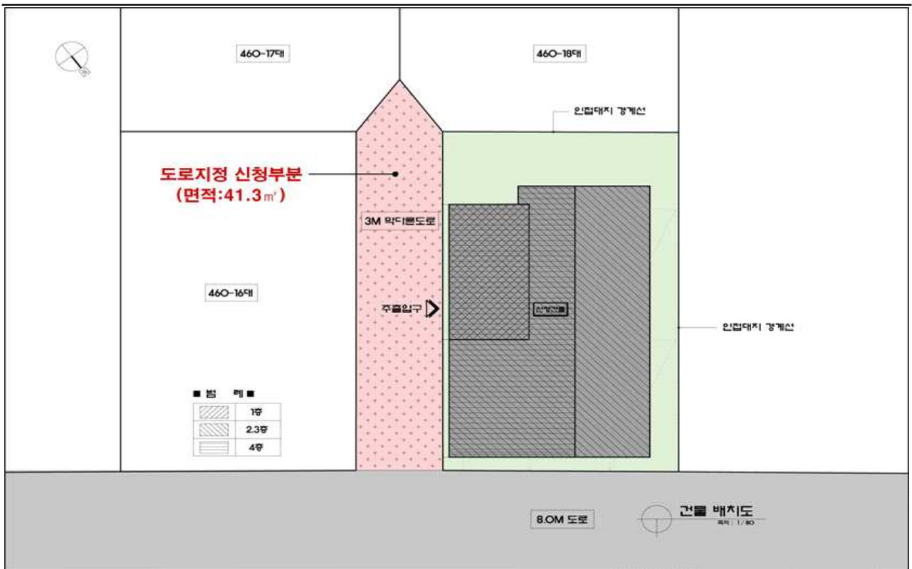
현황도(지적도 첨부)
